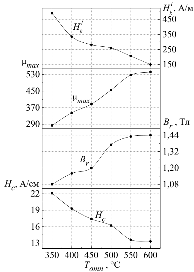
Рисунок 3.10 – Зависимости коэрцитивной силы, остаточной магнитной индукции, максимальной магнитной проницаемости и критического поля, определяемого формой петли гистерезиса, от температуры отпуска закаленных образцов из стали 7Х3, измеренные с помощью магнитоизмерительного комплекса Remagraph С-500
