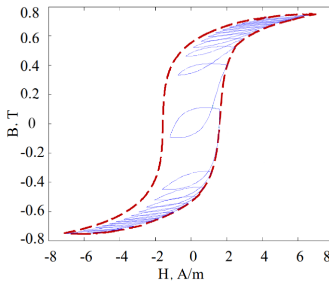
Рисунок 1.1 – Петля гистерезиса перемагничиваемого ферромагнитного материала при смешении частот ([83])
