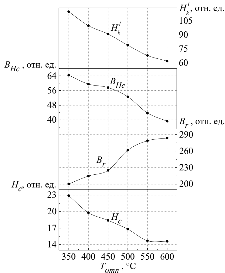
Рисунок 3.11 – Зависимости коэрцитивной силы, остаточной магнитной индукции, индукции коэрцитивного возврата и критического поля, определяемого формой петли гистерезиса, от температуры отпуска закаленных образцов из стали 7X3, измеренные с помощью программно-аппаратной системы DIUS-1.21M
