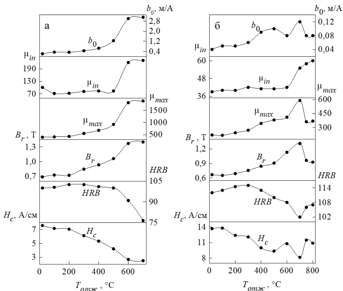
Рисунок 5.1 Зависимости магнитных свойств и твердости от температуры отжига стали 20Г (а) и 70Г (б)
