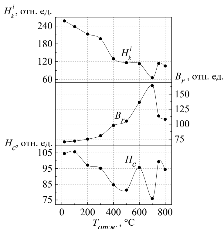
Рисунок 3.15 – Зависимости магнитных свойств от температуры отжига холоддеформированных образцов стали 70Г по результатам локальных магнитных измерений с помощью АПС DIUS-1.21M
