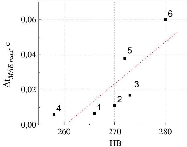
Рисунок 5.14 – Зависимость временного сдвига максимума магнитоакустической эмиссии от твердости исследуемых образцов стали 20ХН2М после прокатки и правки
