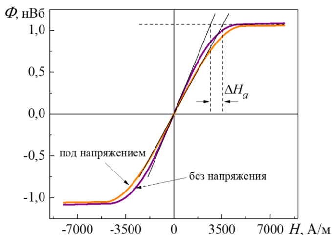
Рисунок 3.1 – Приращение поля анизотропии H_a под действием упругих деформаций ([186])
