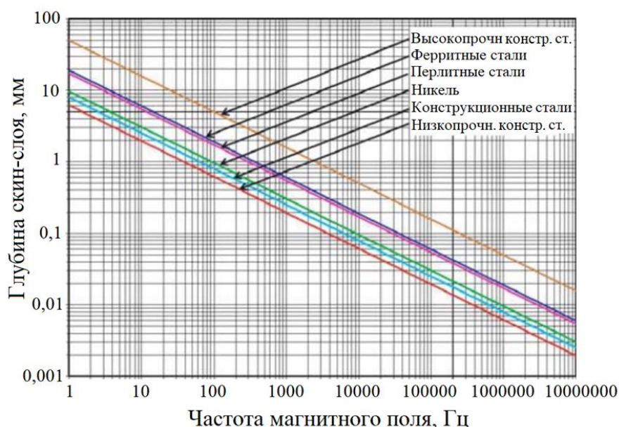
Рисунок 1.3 – Зависимости глубины скин-слоя от частоты перемагничивания для различных классов сталей и никеля ([136])
