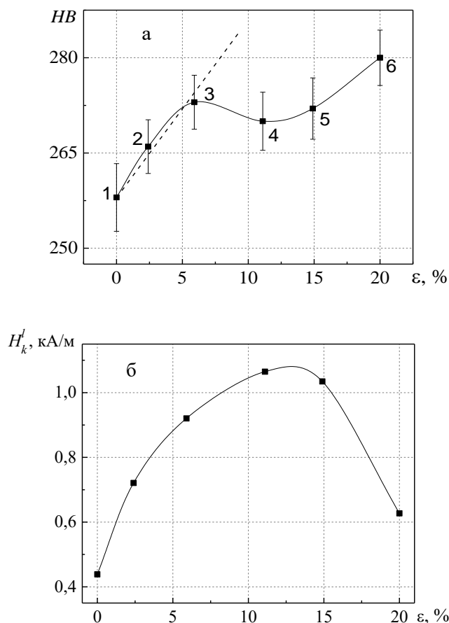
Рисунок 3.7 – Зависимости твердости стальных пластин после пластической деформации прокаткой (а), и критического поля H_k^l (б) от степени пластической деформации образцов стали 20ХН2М
