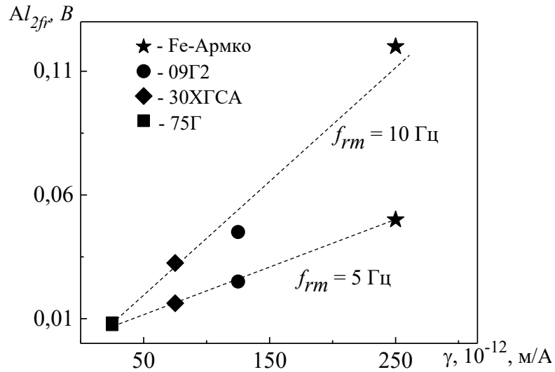
Рисунок 4.12 – Зависимость амплитуды гармоники l_{2fr} от магнитострикционной чувствительности \gamma отожженных сталей и Fe-АРМКО
