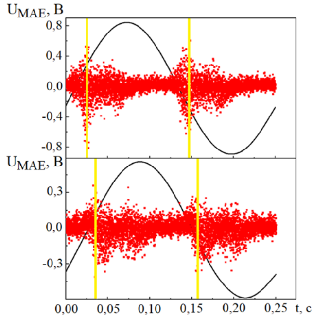
Рисунок 4.14 – Фрагменты оцифрованных осциллограмм переменного магнитного поля (●) и магнитоакустической эмиссии (■), отожденного при 700 °С (вверху) и при 200 °С (внизу) образцов из стали 70Г
