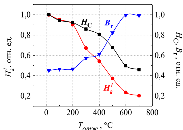
Рисунок 3.14 – Зависимости коэрцитивной силы, остаточной магнитной индукции и критического поля, определяемого формой петли гистерезиса в относительных единицах, от температуры отжига образцов из холоддеформированной стали 20Г, измеренные с помощью программно-аппаратной системы DIUS-1.21M
